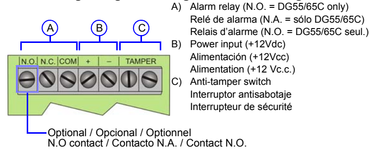
Figure/Figura 4 PCB Overview / Vista General / Vue d'ensemble
