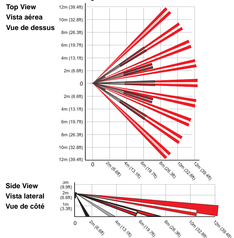
Figure 2: DG55/DG65 Beam Pattern / Estructura de Haces / Diagramme de faisceau
